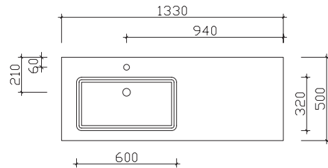
Width 1330 mm BLE015F13302
