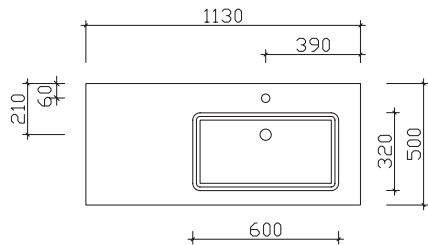
Width 1130 mm BRE015F11302
