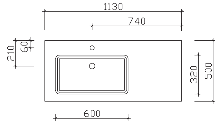
Width 1130 mm BLE015F11302
