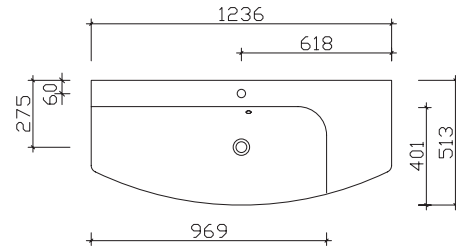
Width 1236 mm RD-MMWTR65-1236
