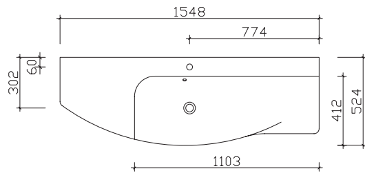
Width 1548 mm RD-MMWTR65-1548
