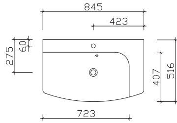
Width 845 mm RD-MMWTR65-845
